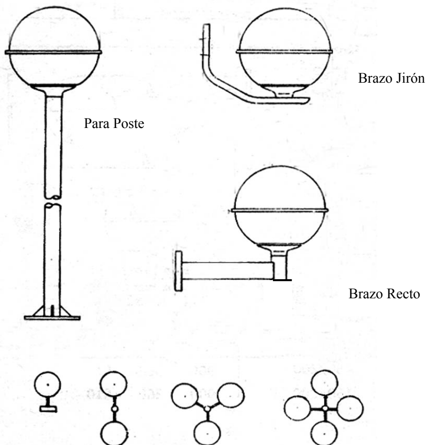
Vista de Elevación
